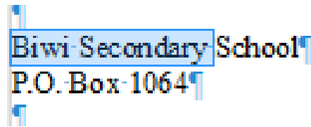
Fig. 1.14 Highlighted text
